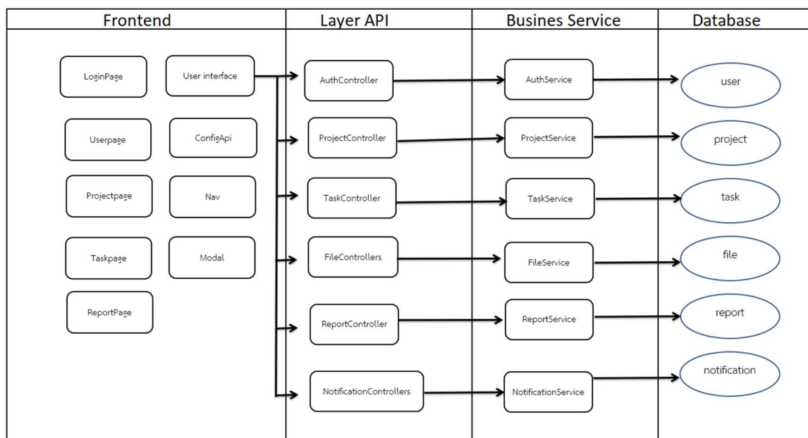
ภาพ ค-1 Building block and Diagrams
