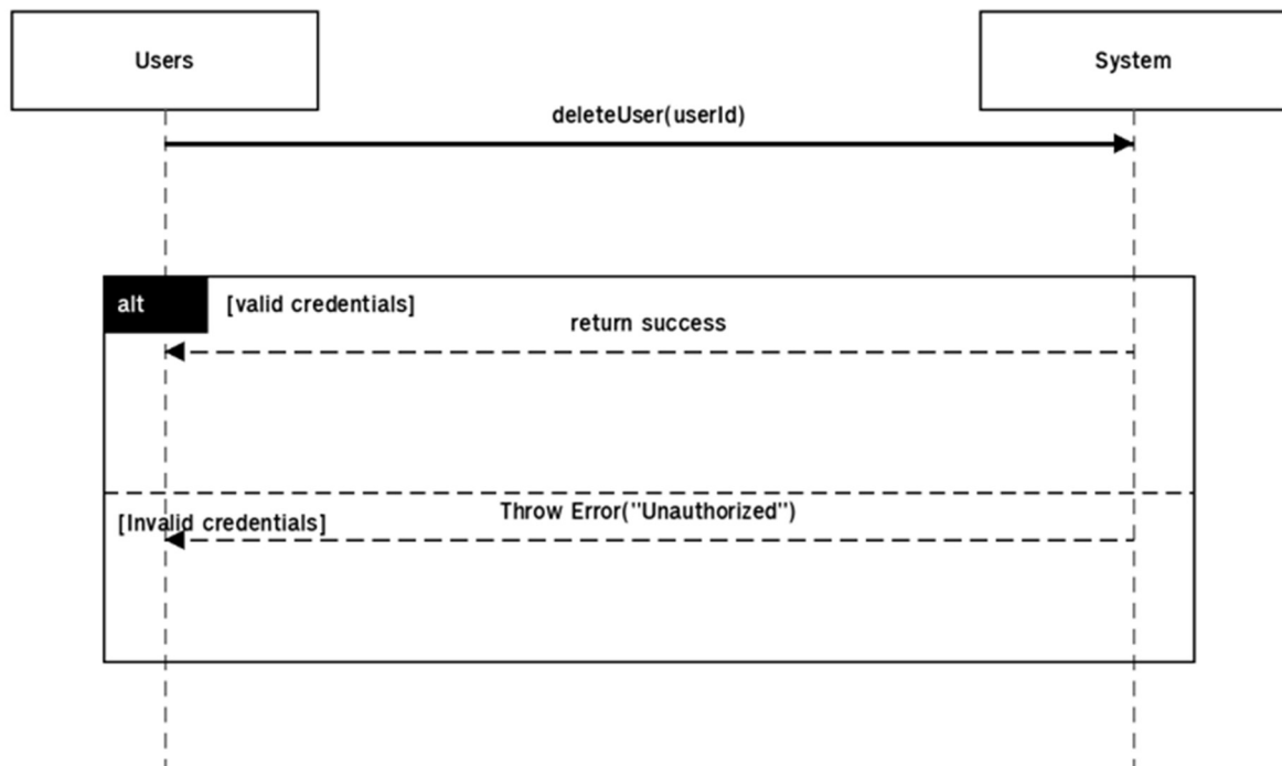
ภาพ ค-7 Sequence Diagram IDSQ-TAT-02
