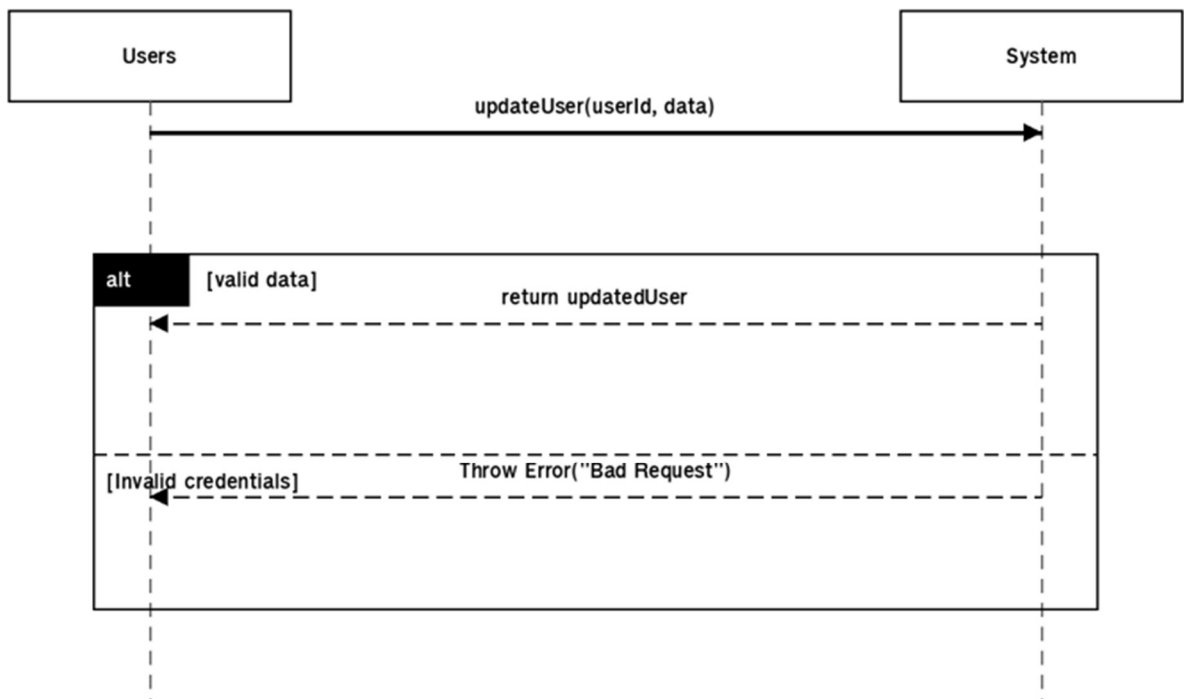
ภาพ ค-8 Sequence Diagram IDSQ-TAT-03
