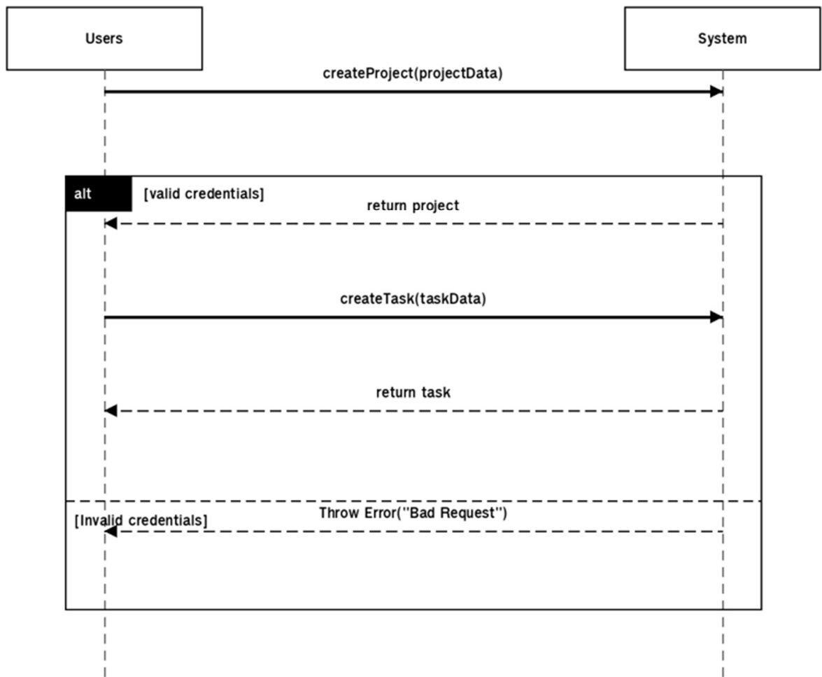
ภาพ ค-9 Sequence Diagram IDSQ-TAT-04
