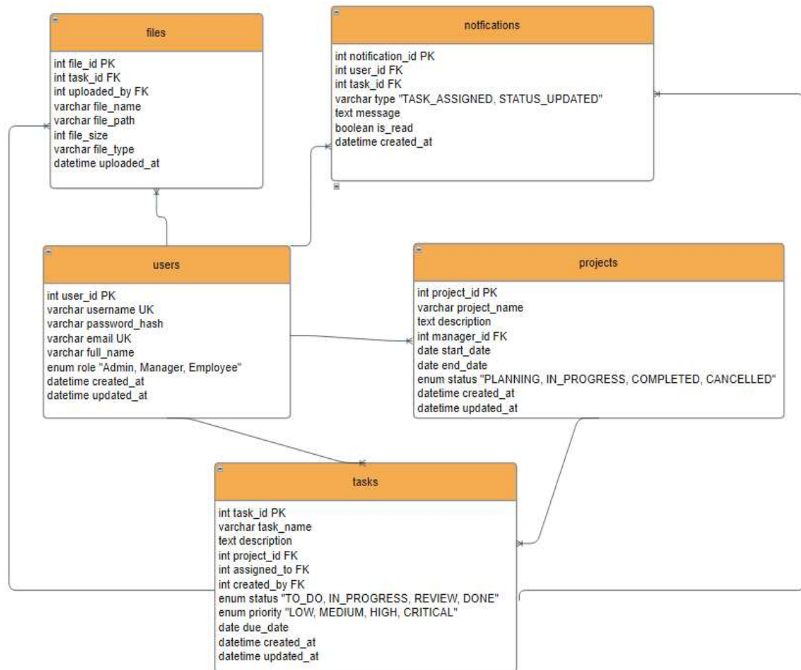
ภาพ ค-11 ER Diagram
