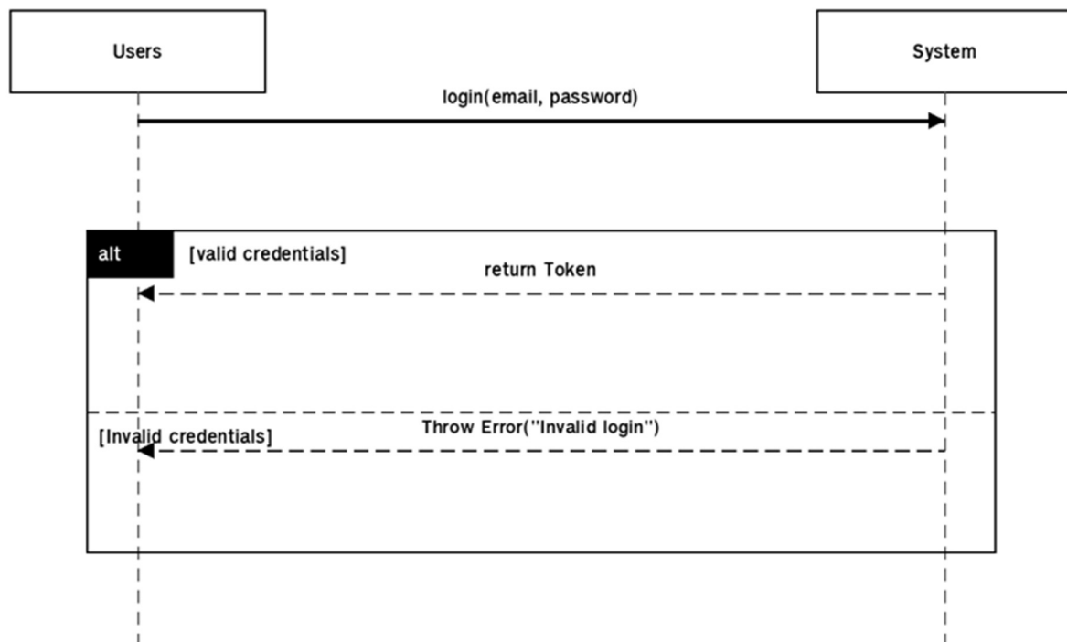
ภาพ ค-6 Sequence Diagram IDSQ-TAT-01
