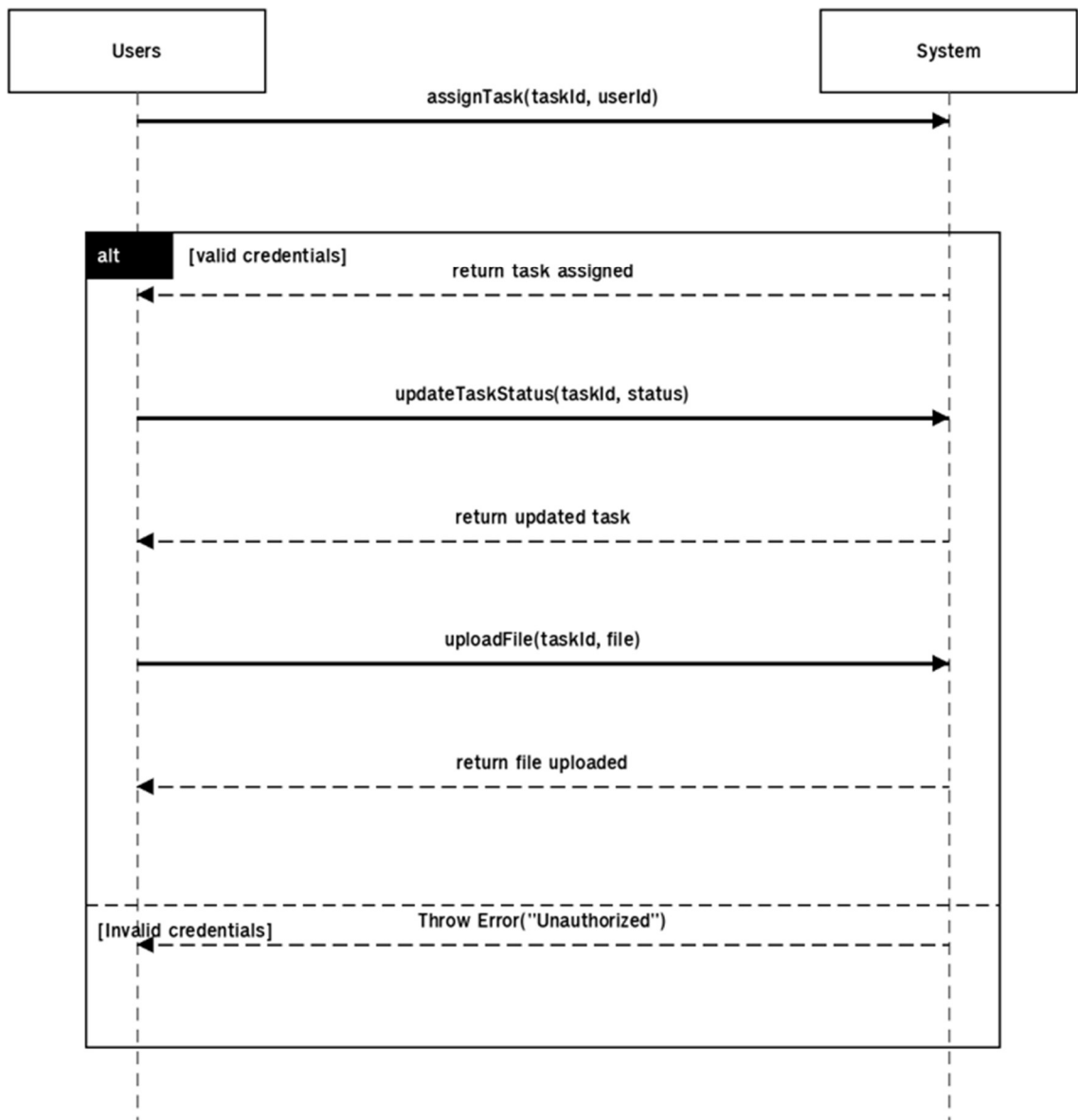
ภาพ ค-10 Sequence Diagram IDSQ-TAT-05
