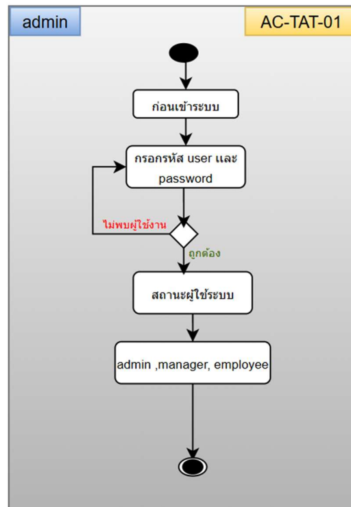
ภาพ ค-4 Activity ID AC-TAT-01
