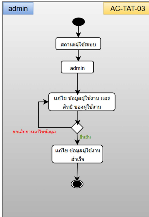
ภาพ ค-6 Activity ID AC-TAT-03
