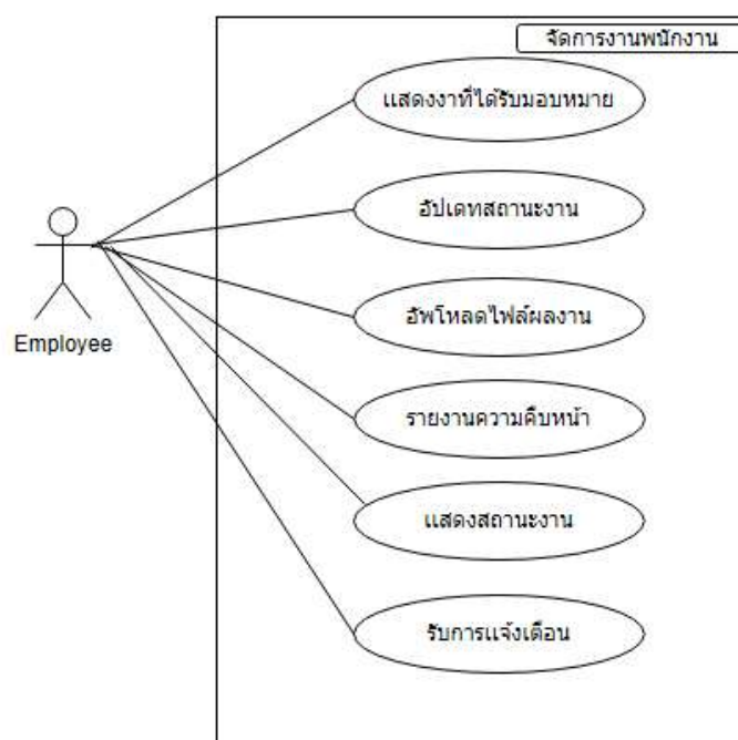
ภาพ ค-4 Use Case Diagram แสดงภาพรวมของพนักงาน
